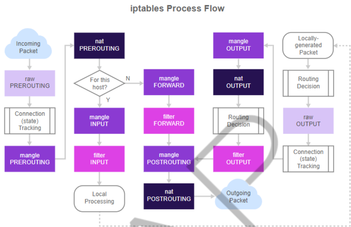
Figura 17 – Fluxo de Processo do iptables Fonte: Phil Hagen (2014)
